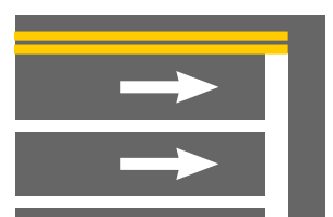
H 4 Marcas transversales Línea de detención
